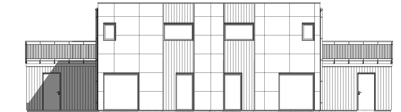
FASAD A3 1:100
